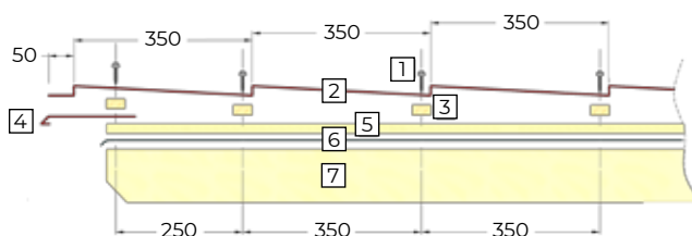
2. ábra Cserepeslemez klasszikus beépítési módja fa fedélszerkezetre
